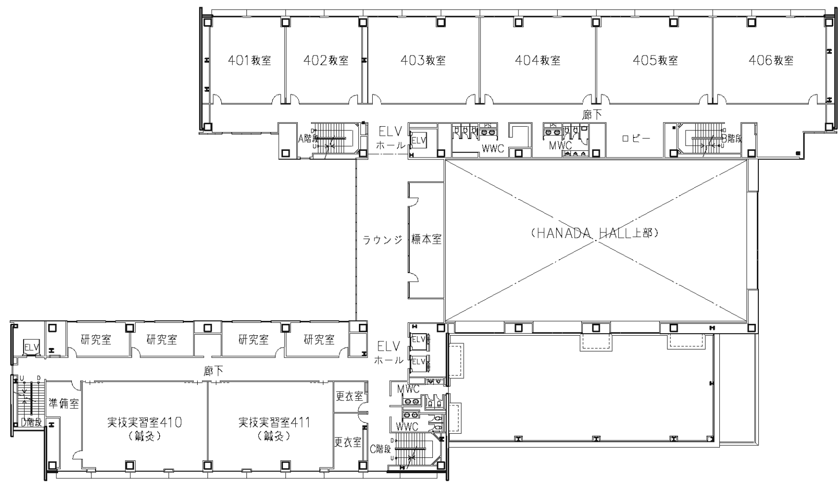
4階平面図
